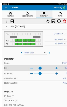
Parameter-Screen mit visualisiertem Erfassungsfeld bei den Sensor-Einstellungen.
